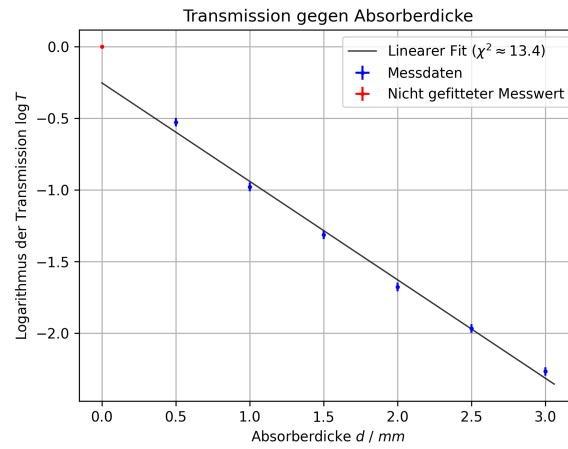
Abbildung 22: Linearer Fit des Transmissionsgrads T gegen Absorberdicke d (Molybdän-Röhre, U = 35 kV, ohne Zirkoniumfilter)
