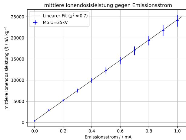
Abbildung 15: mittlere Ionendosisleistung \langle j \rangle in Abhängigkeit des Emissionsstroms I (Molybdän-Röhre, I = 35 \text{ kV} )
