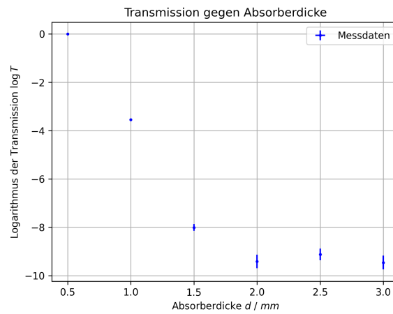
Abbildung 23: Transmissionsgrad T gegen Absorberdicke d (Molybdän-Röhre, U = 35 kV, mit Zirkoniumfilter)
