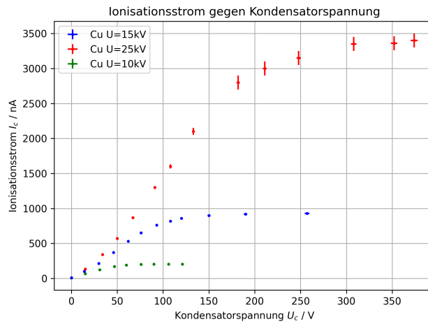
Abbildung 14: Ionisationsstrom I_C des Kondensators in Abhängigkeit der Kondensatorspannung U_C für drei verschiedene Röhrenspannungen (Kupfer-Röhre, I = 1 mA)
