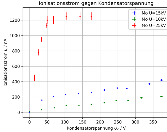
Abbildung 12: Ionisationsstrom I_C des Kondensators in Abhängigkeit der Kondensatorspannung U_C für drei verschiedene Röhrenspannungen (Molybdän-Röhre, I = 1 \text{ mA} )
