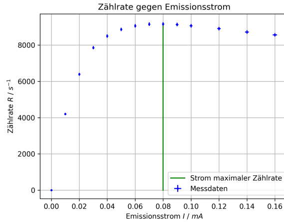
Abbildung 21: Zählrate R gegen Emissionsstrom I (Kupfer-Röhre, U = 35 kV)
