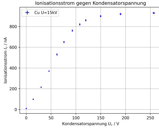
Abbildung 13: Ionisationsstrom I_C des Kondensators in Abhängigkeit der Kondensatorspannung U_C für Röhrenspannung U = 15 kV (Kupfer-Röhre, I = 1 mA)
