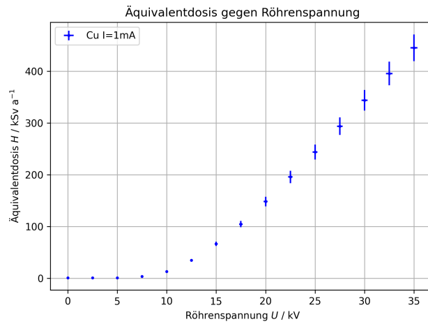
Abbildung 18: Äquivalentdosis H pro Jahr in Abhängigkeit der Röhrenspannung U (Kupfer-Röhre, I = 1 mA)
