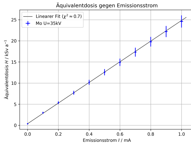
Abbildung 17: Äquivalentdosis H pro Jahr in Abhängigkeit des Emissionsstroms I (Molybdän-Röhre, U = 35 kV)
